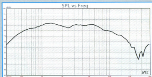
FIGURE 10: EM 1308 on-axis response.
